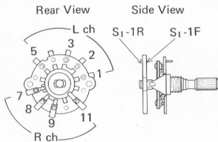
S 1 : FUNCTION switch
